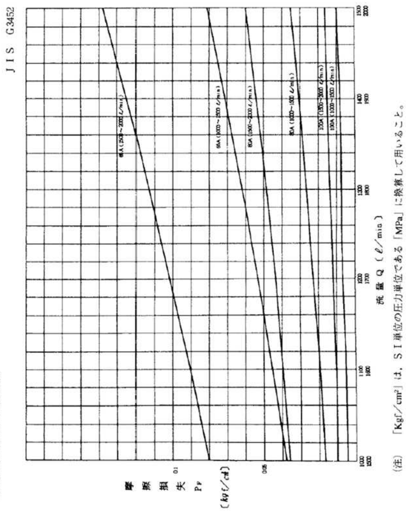
図3-7 等価管長1 m当りの摩擦損失
