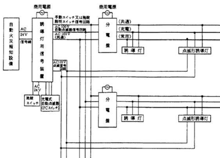
圖16-23 機器結線圖
