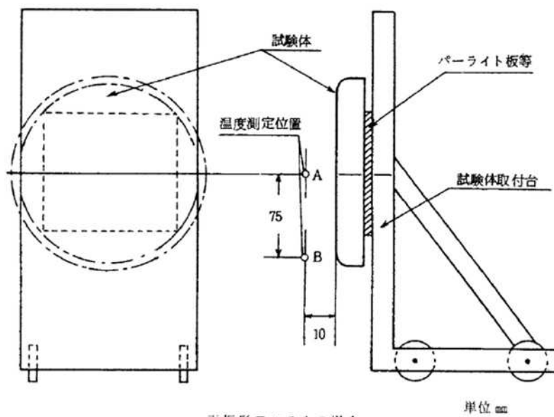
平板形アンテナの場合
