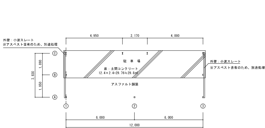
平面図 S=1/100
