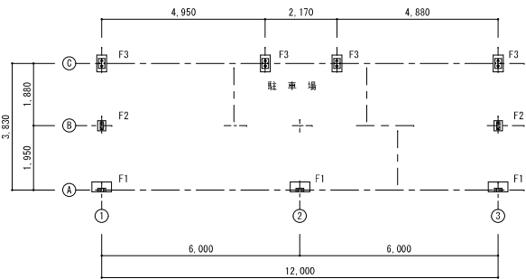
基礎伏図 S=1/100
