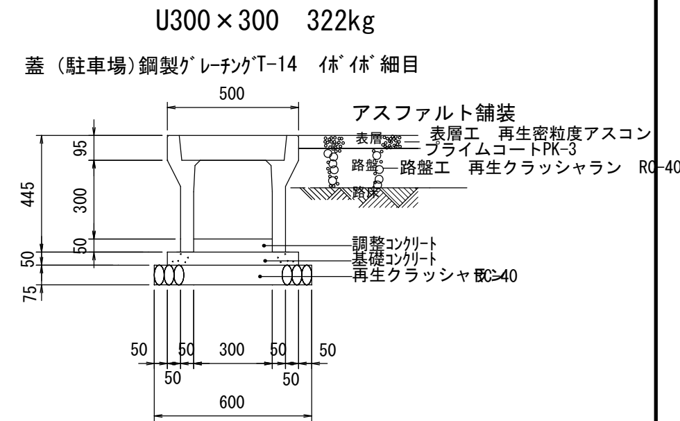
自由勾配側溝 1/20
