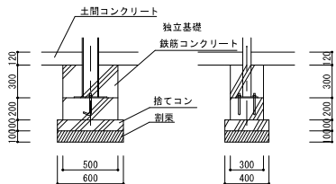
F3基礎構造図 1/30
