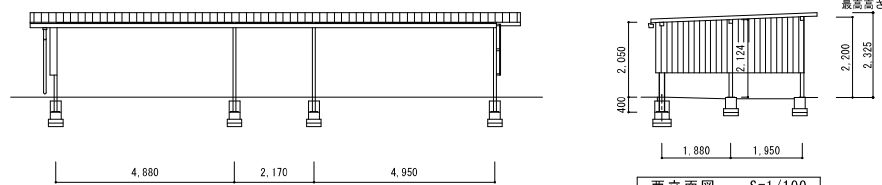
西立面図 S=1/100
