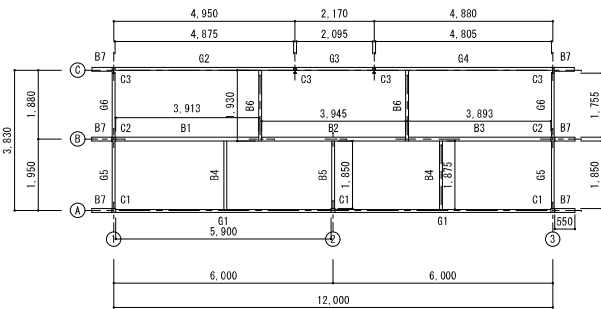
梁伏図 S=1/100
