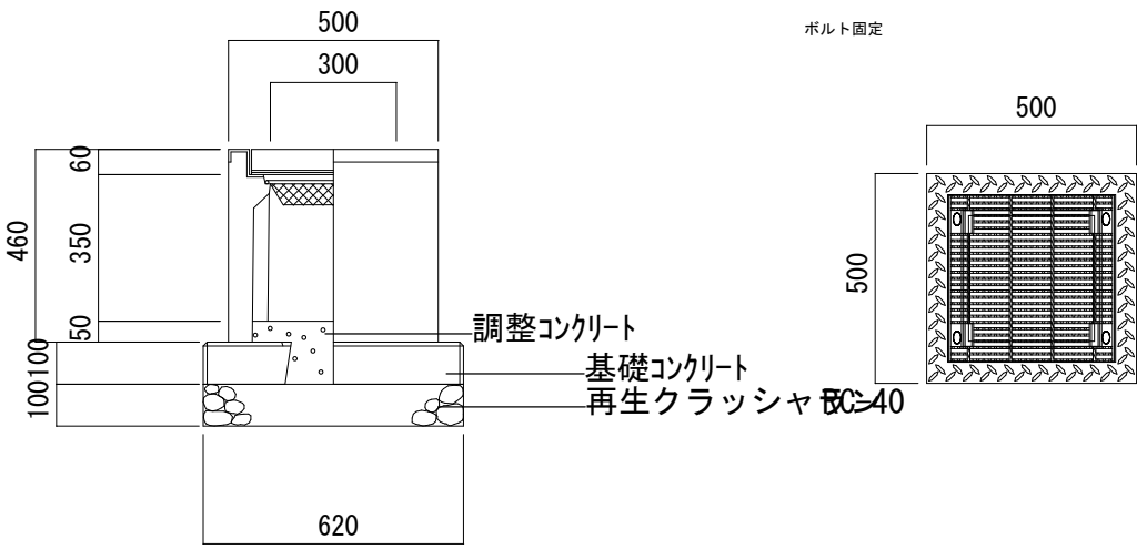
集水樹 G1 A S 型 可変側溝用樹 (スタンダード)1/20
