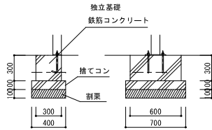
F1基礎構造図 1/30
