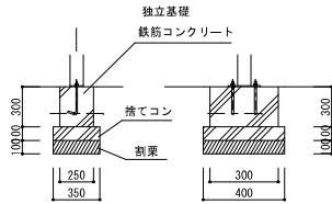
F2基礎構造図 1/30
