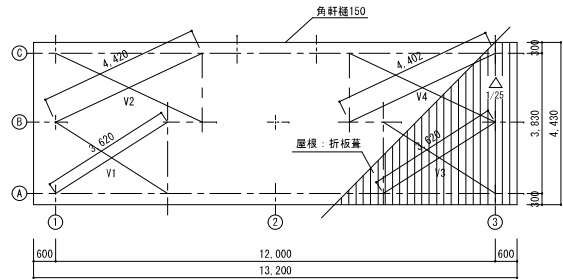
屋根伏図 S=1/100
