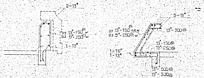
配筋図 6c 1/30
