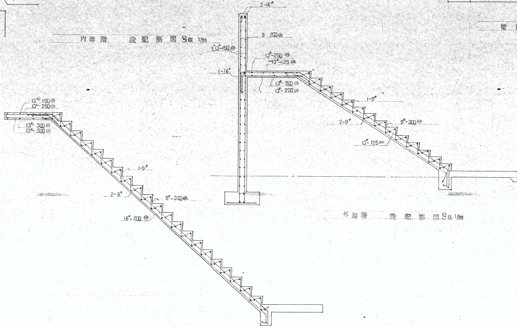
外部階段配筋図 S&1/80
