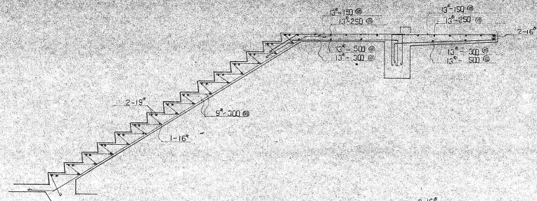
内部階段配筋図 S&1/80
