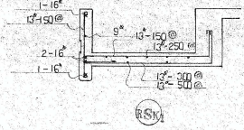
壁配筋図 S&1/80
