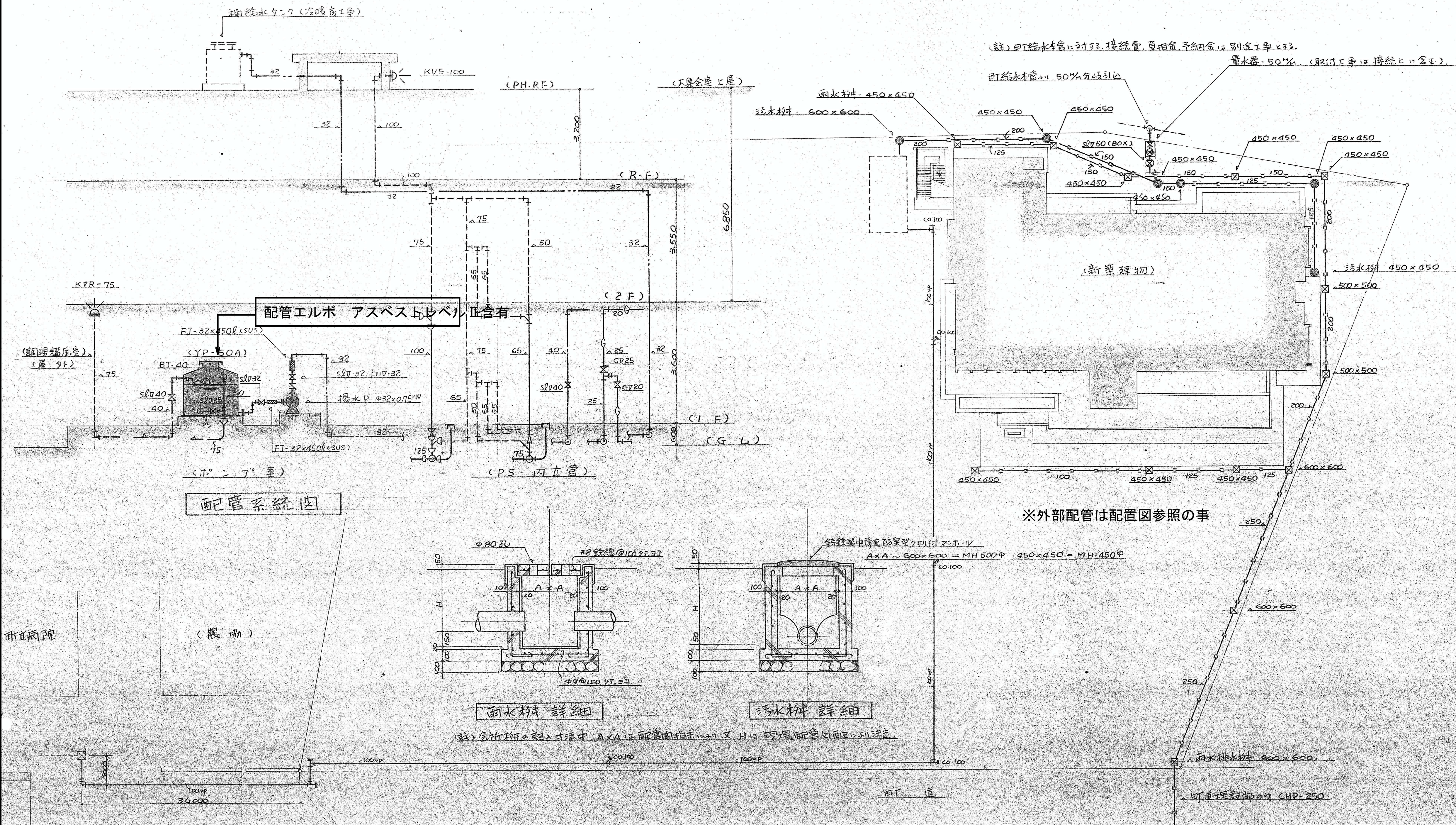
屋外配管図 1/200
